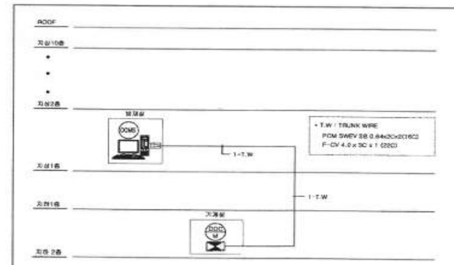
자동제어 시스템 구성도
